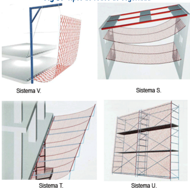
Fig 5: Tipos de redes de seguridad
